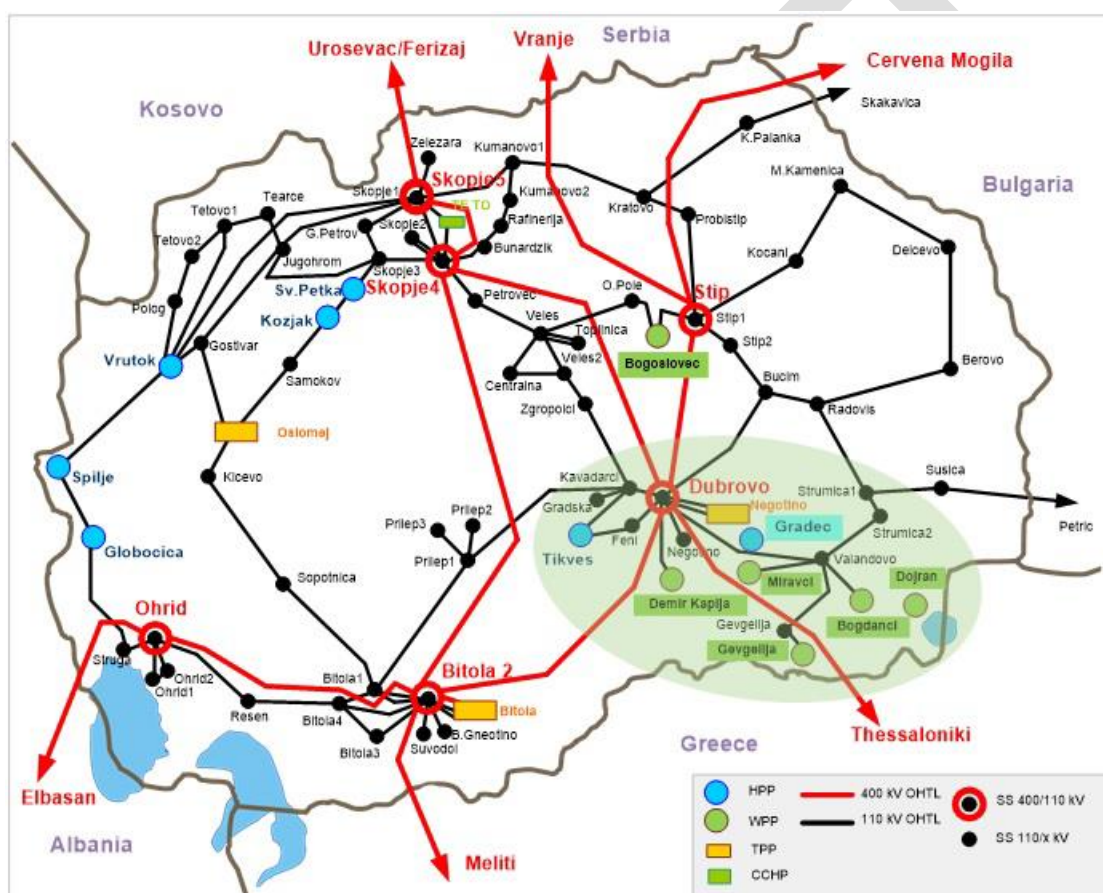
Слика 2.1: Македонската преносна мрежа и проектна област, топологија на среден рок
